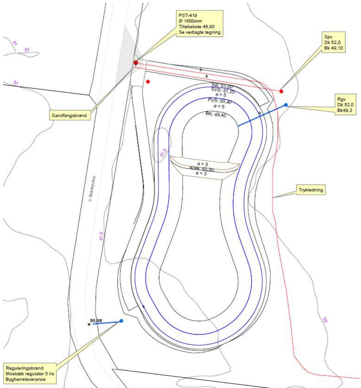
Regnvandsbassinets udformning
